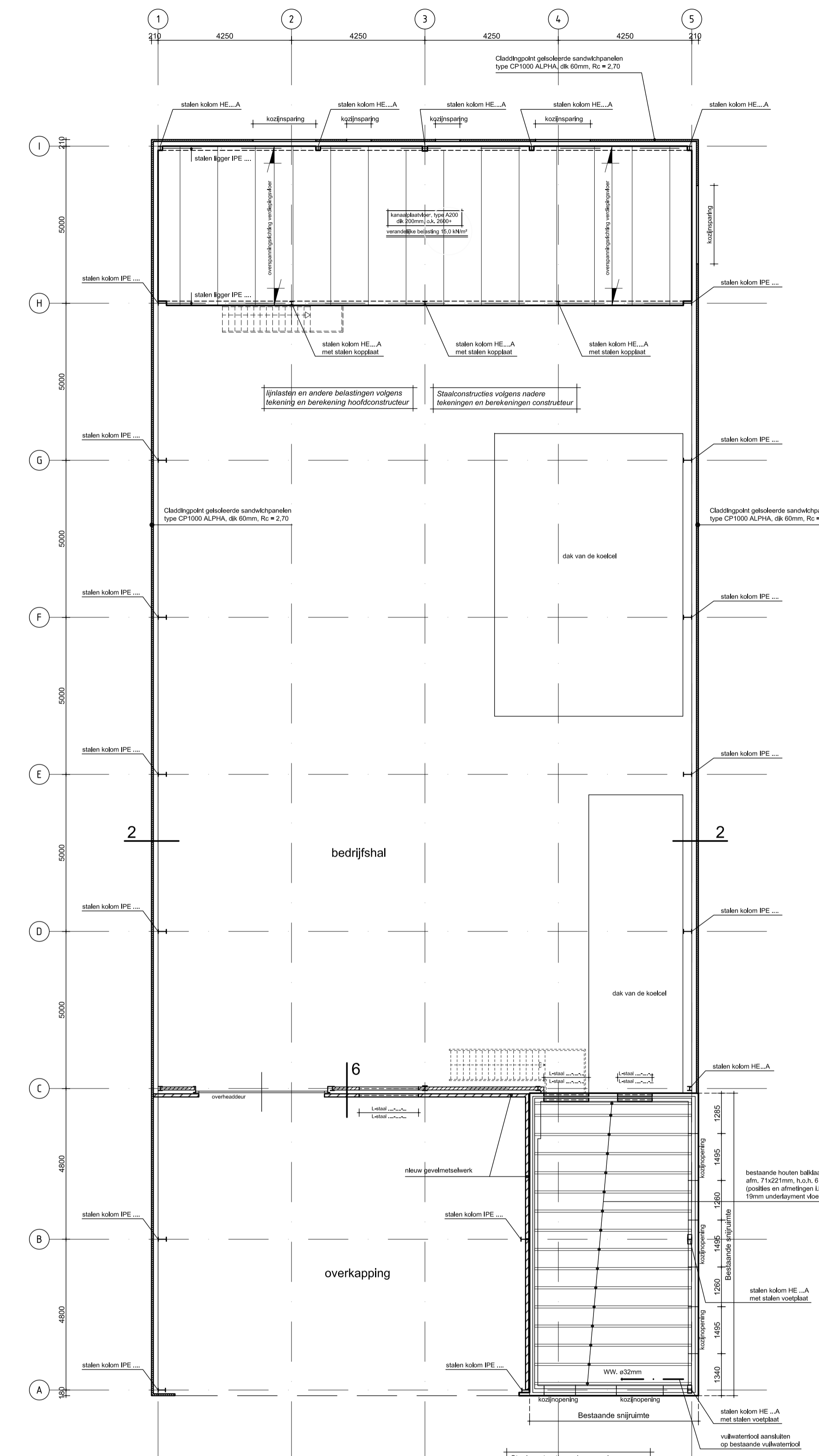
1e verdiepingvloer stramien H en I 1:50
