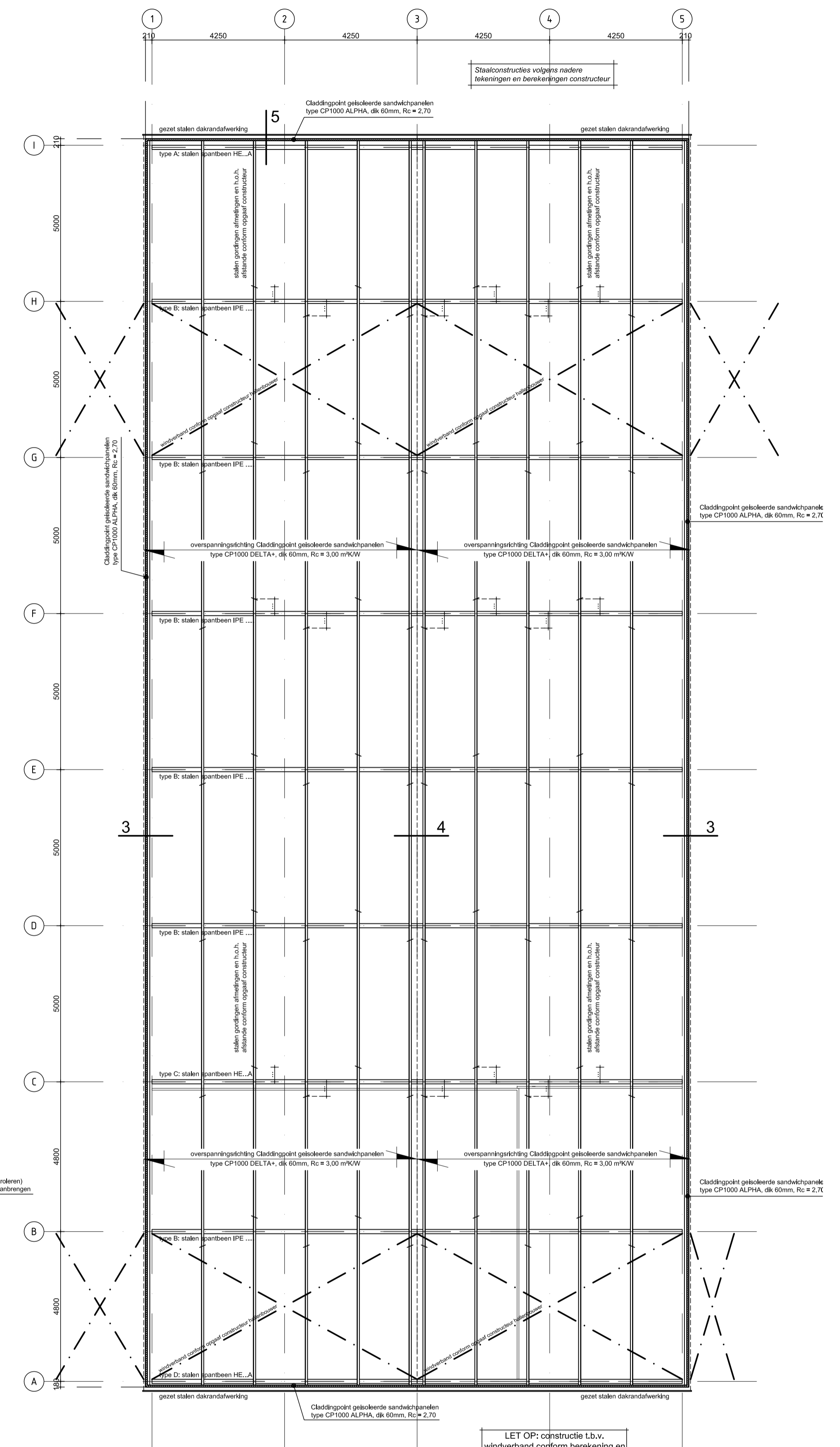
Staal- en dakconstructie 1:50
